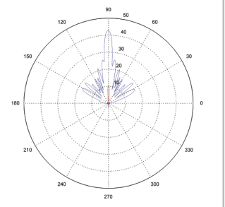
6.0 Ghz H-Plane and E of H-plane
