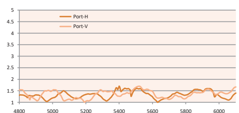
Antenna VSWR 5400-6700 MHz
