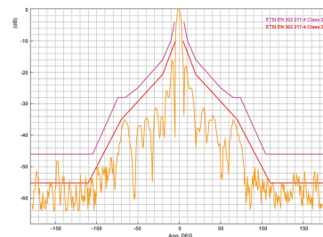
6.5 GHz H-Plane
