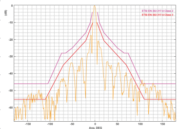
6.5 GHz E-Plane
