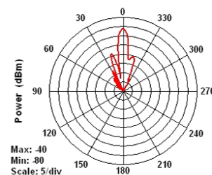
5.5 Ghz H-Plane and E of H-plane
